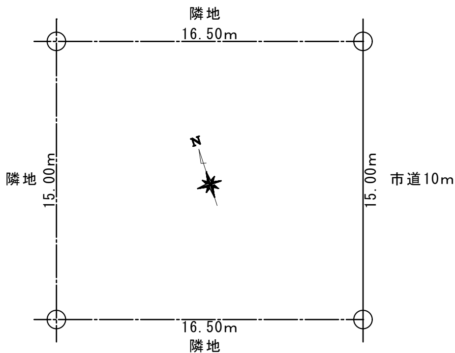
配置図 1/200
