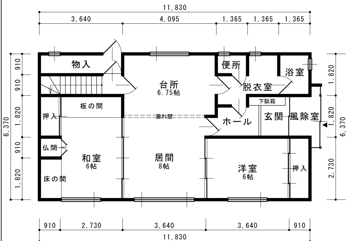
1階平面図 1/100
