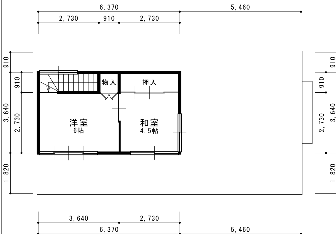
2階平面図 1/100
